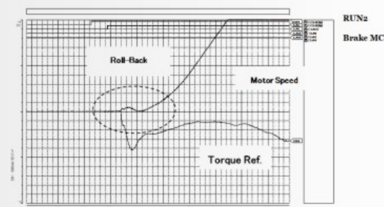
Diagrama de arranque de enlace ascendente del ascensor tradicional
