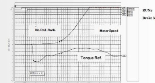
Diagrama de arranque de enlace ascendente de ascensor libre de sensibilidad
